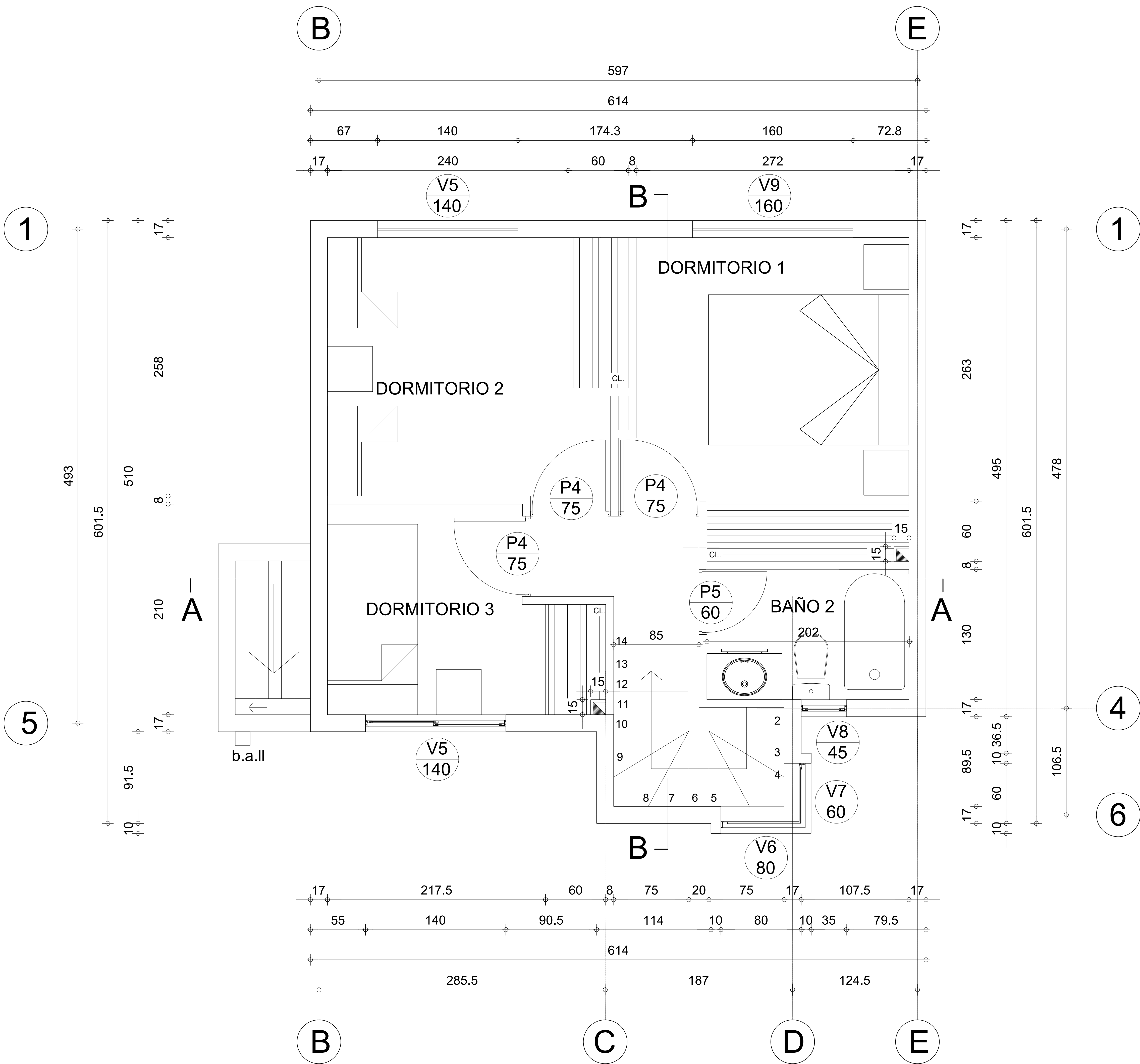
PLANTA SEGUNDO PISO ESCALA 1:50
